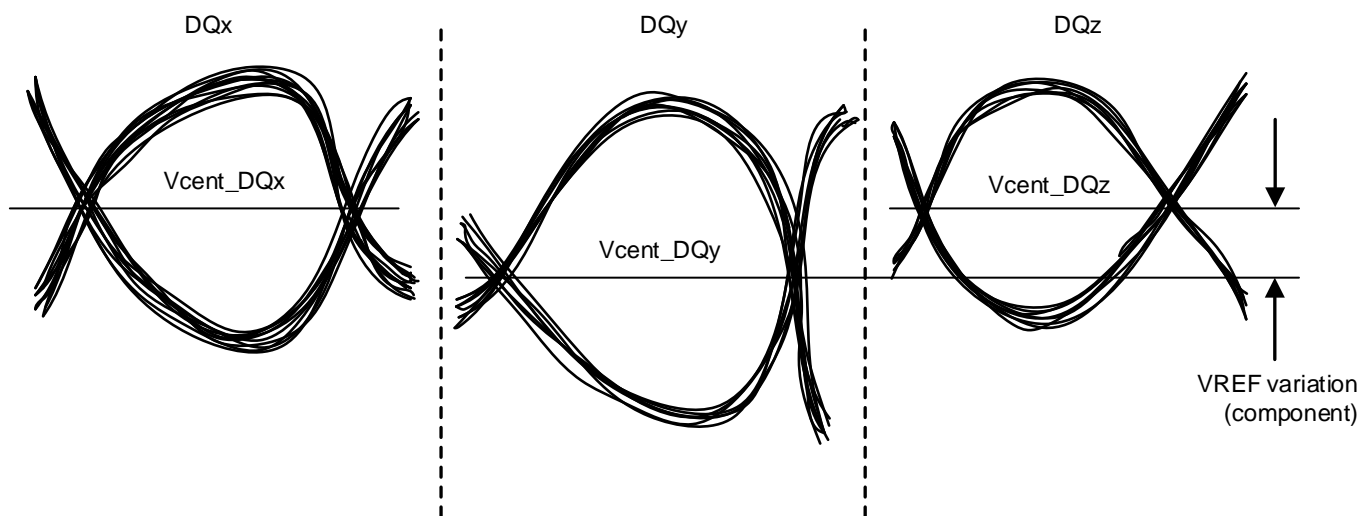
Figure 8-9 Across Pin VREF DQ Voltage Variation
