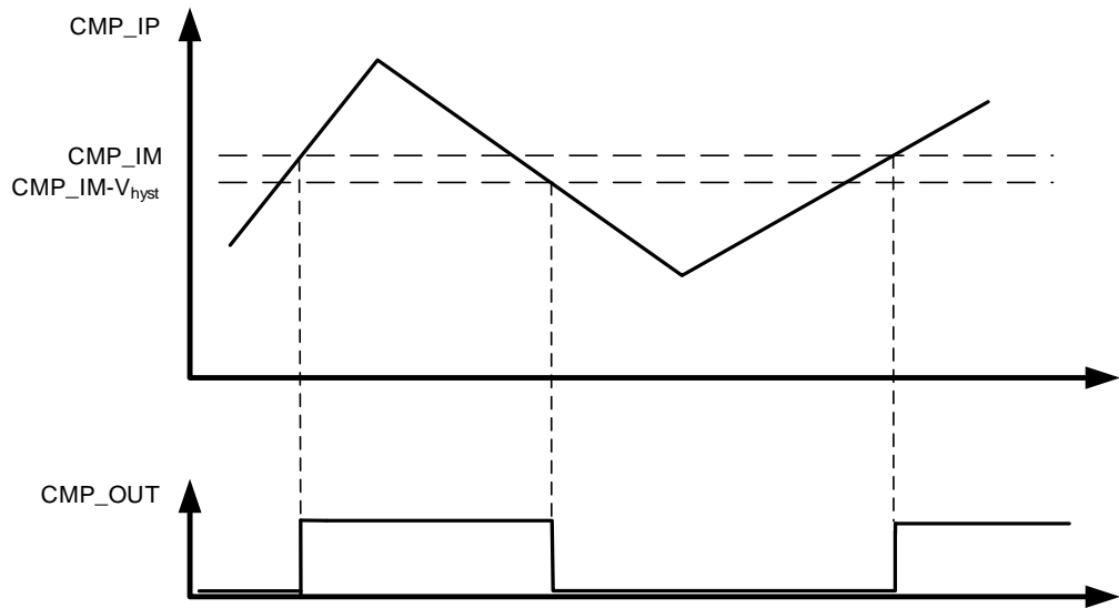
图 22-2. 比较器迟滞
