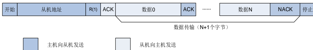
图 20-6. 7 位地址的 I2C 通讯流程（主机接收）
