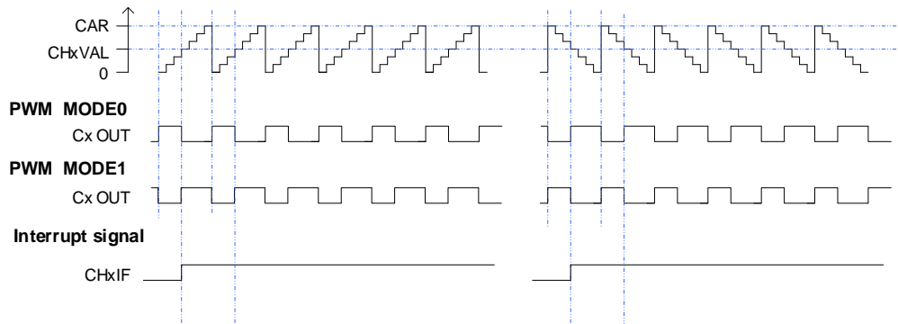
图 18-54. CAPWM 时序图
