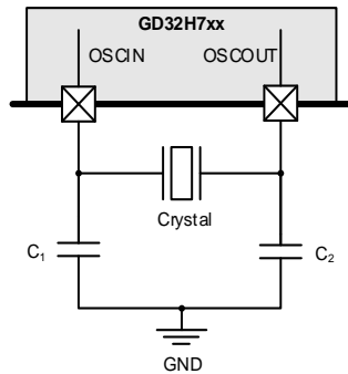
图 2-22. HXTAL 外部时钟电路
