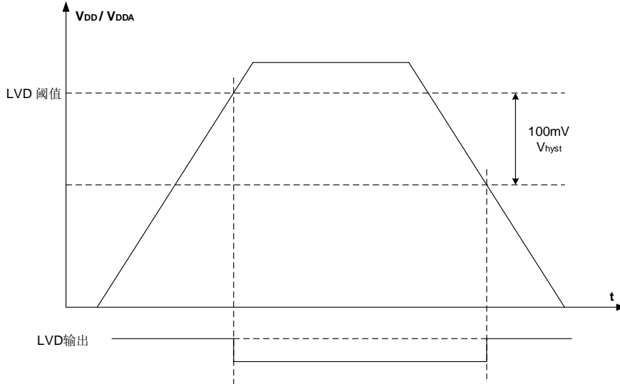
图 2-16. LVD 阈值波形图
