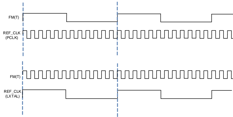
图 2-29. 测量方式
