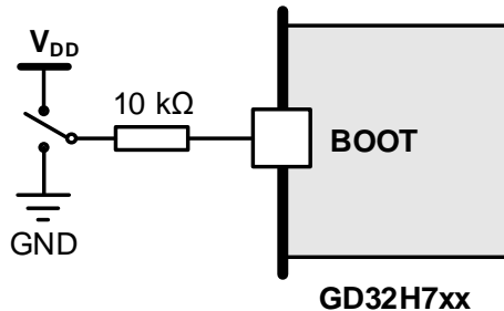
图 2-25. 推荐 BOOT 电路设计
