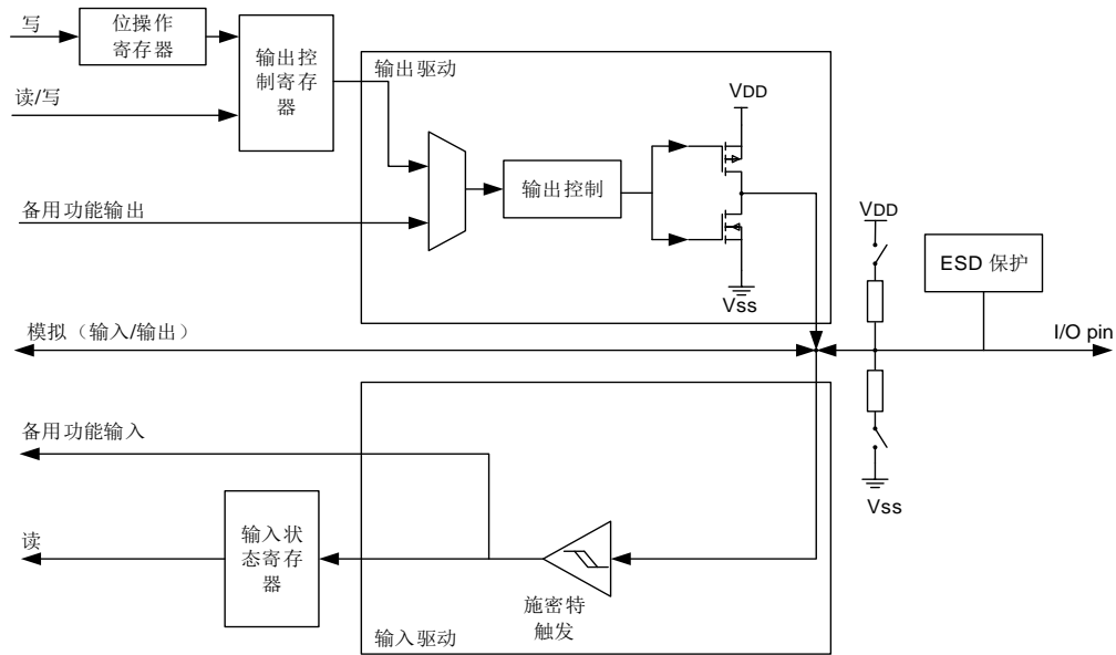
图 2-26. 标准 IO 的基本结构
