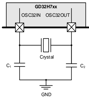
图 2-24. LXTAL 外部时钟电路
