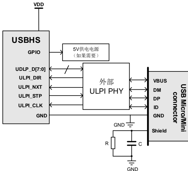
图 2-32. 使用外部 ULPI PHY 的连接示意图
