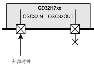
图 2-24. LXTAL 外部时钟电路
