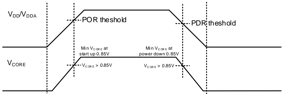
图 2-9. 旁路模式上电时序图
