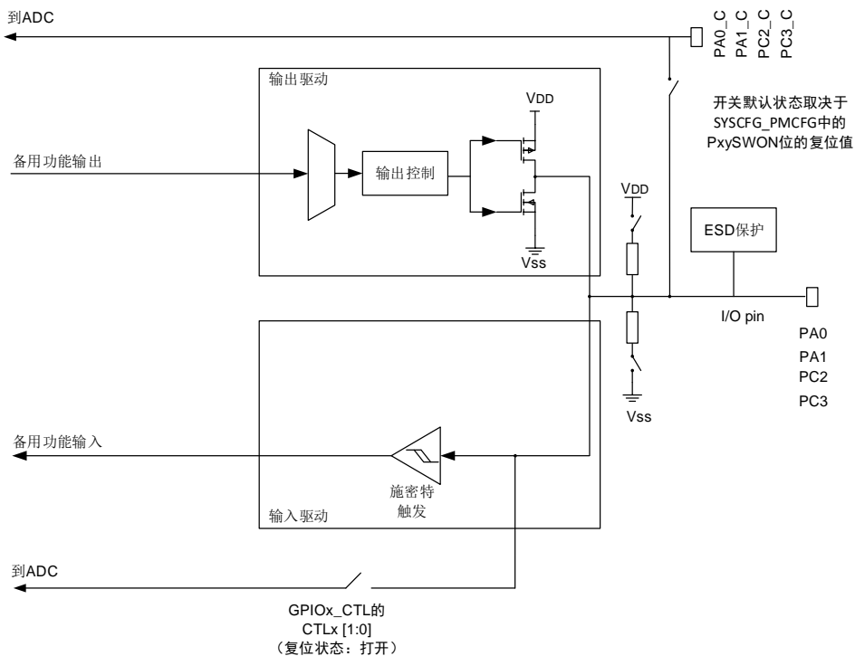
图2-28. ADC 的模拟配置
