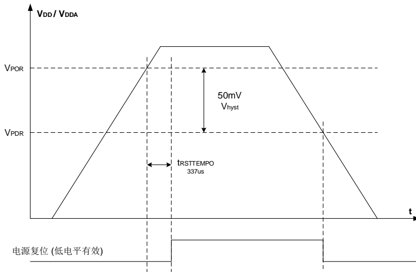
图2-14. 上电 / 掉电复位波形图
