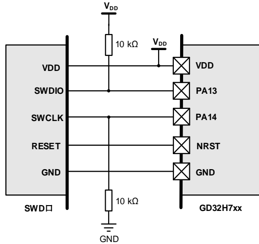
图 2-35. 推荐 SWD 接线参考设计
