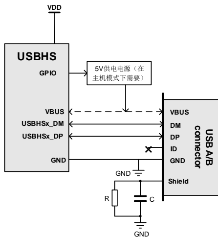
图 2-30. 在主机或设备模式下连接示意图
