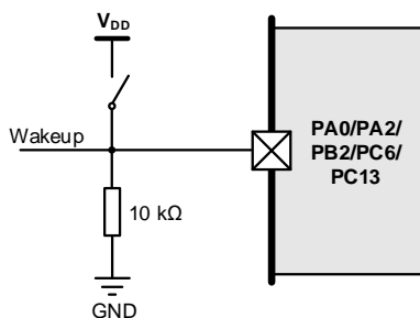
图 2-33. 推荐 Standby 外部唤醒引脚电路设计
