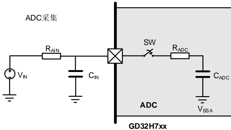
图 2-27. ADC 采集电路设计
