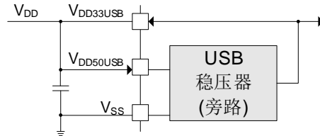
图 2-11. USB 稳压器旁路时连接示意图
