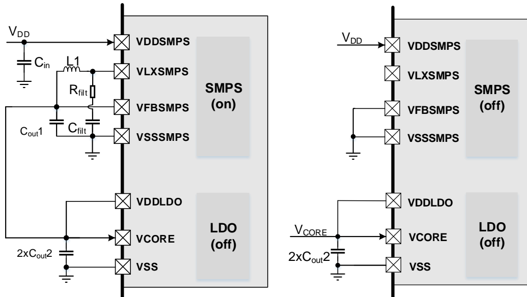
图 2-13. GD32H7xx 系列 SMPS 降压稳压器推荐设计
