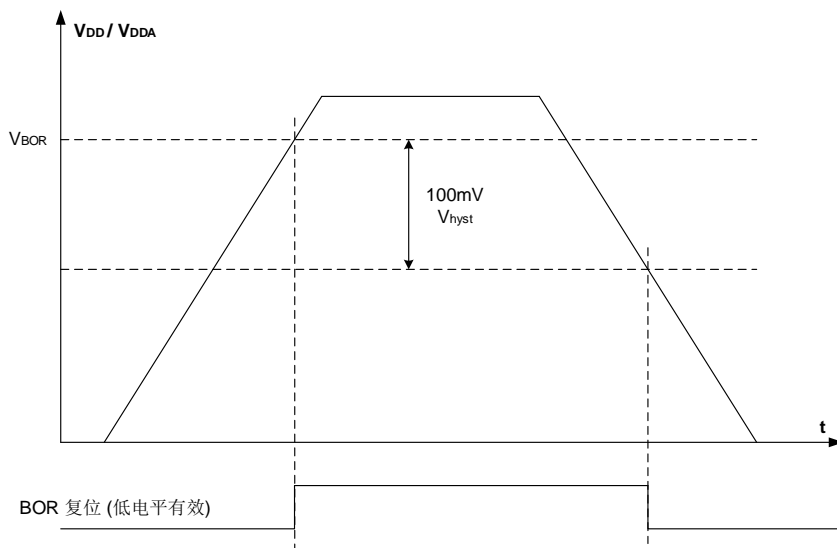
图2-15. BOR波形图
