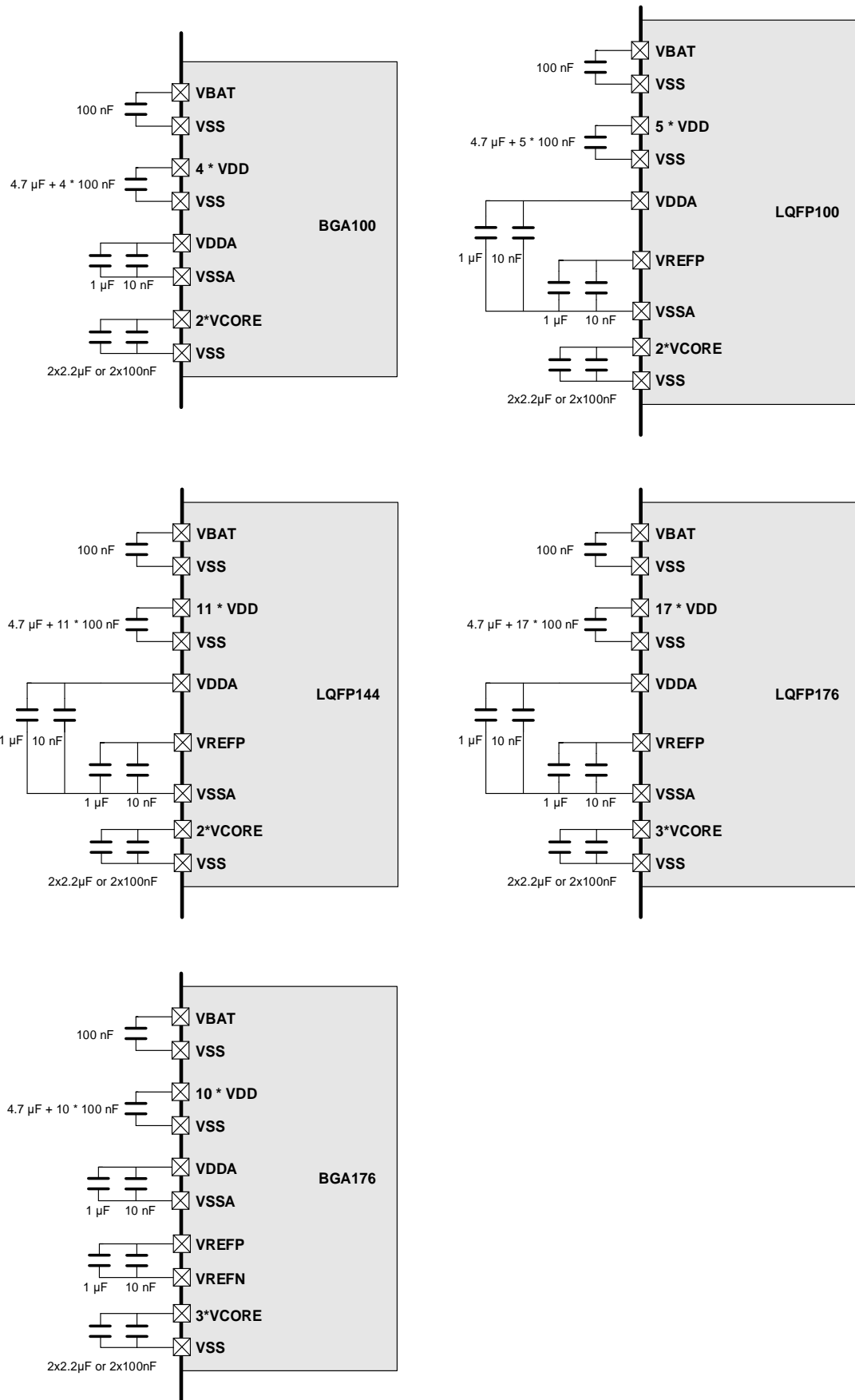
图 2-12. GD32H7xx 系列推荐供电设计
