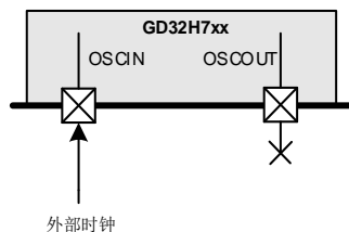
图 2-22. HXTAL 外部时钟电路
