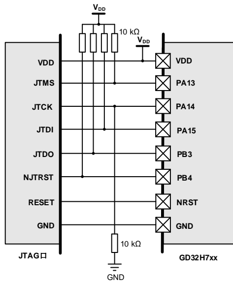
图 2-34. 推荐 JTAG 接线参考设计
