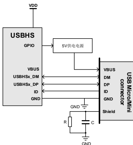
图 2-31. OTG 模式下使用内部嵌入式 PHY 连接示意图
